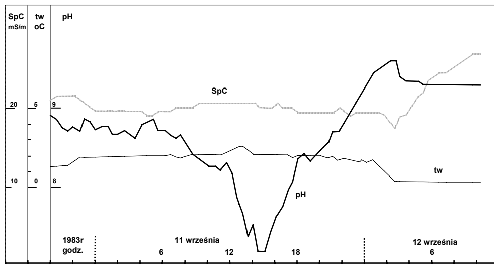
Rys. 4.5.1. Zmiany pH, SpC i t_w (temperatury) wody w rzece lodowcowej Lodowca Werenskiolda po wystąpieniu zjawiska fenowego we wrześniu 1983 roku (Głowacki 1983). Changes of pH, SpC and temperature ( t_w ) of water in a glacial river discharging from Werenskioldebreen in September 1983, after phoen phenomena (Głowacki 1983).
