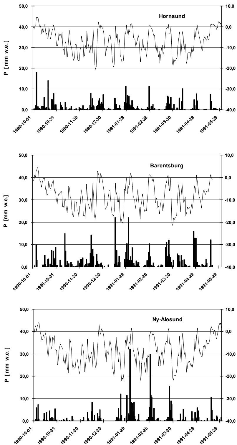
Rys. 4.2.4. Średnie dobowe temperatury powietrza i sumy opadu atmosferycznego na stacjach Hornsund, Barentsburg i Ny-Alesund znajdujących się na zachodnim wybrzeżu Spitsbergenu, w sezonie zimowym 1990/1991 (Głowacki, Pulina 2000). Mean daily air temperatures and precipitation totals at the stations located on the western coast of Spitsbergen: Hornsund, Barentsburg and Ny-Alesund in the winter season of 1990/1991 (Głowacki, Pulina 2000).
