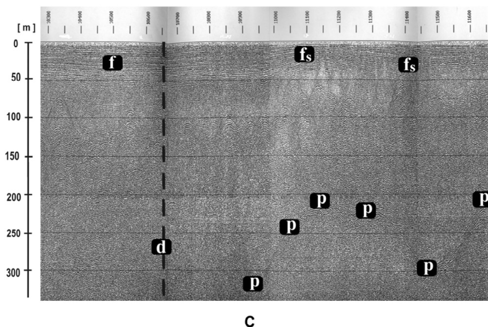
Rys. 4.4.3. Zdjęcie radarowe (częstotliwość 50 MHz) profilu części akumulacyjnej Lodowca Hansa w roku 1998r z zaznaczoną lokalizacją pionowego profilu termicznego (patrz Rys. 3.5 – profil c oraz punkt pomiarowy d; warstwy firnu – f; zaburzone ułożenie warstw firnu – f_s ; podłoże lodowca – p). Radar measurements (50 MHz frequency) in the profile of Hansbreen (accumulation part) in 1998 with marked location of the vertical thermic profile (see Fig. 3.5 – profile c and measuring point d; f – firn layer; f_s – firn dislocation layers; p – bedrock).
